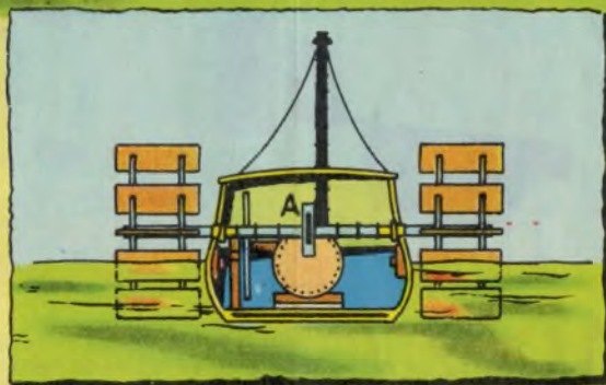
Coupe transversale du Pyroscaphe.
